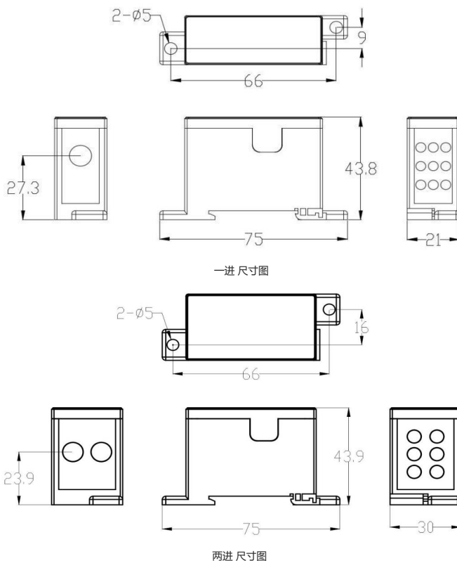
一进尺寸图
